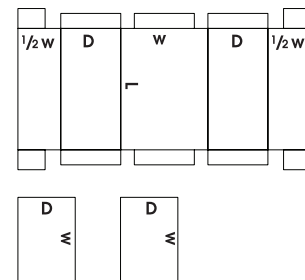
0606A Bliss Style Container
